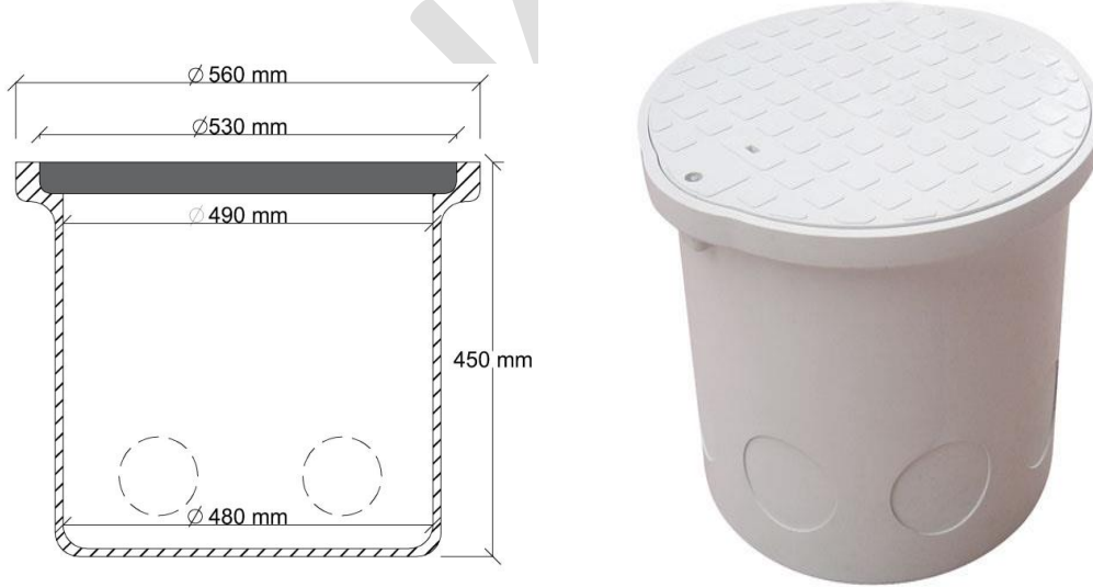
Şekil 4. TİP 20A-B Kompozit Silindir Ek Odaları
