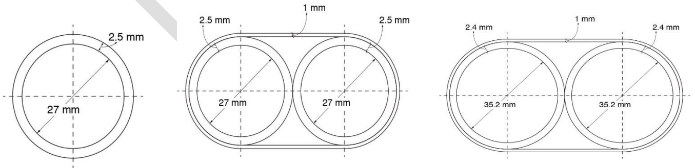
Şekil 1. 32 mm HDPE 12,5 ATÜ Boru & 2x40 mm HDPE 12,5 ATÜ Boru & 2x40 mm HDPE 10 ATÜ Boru
