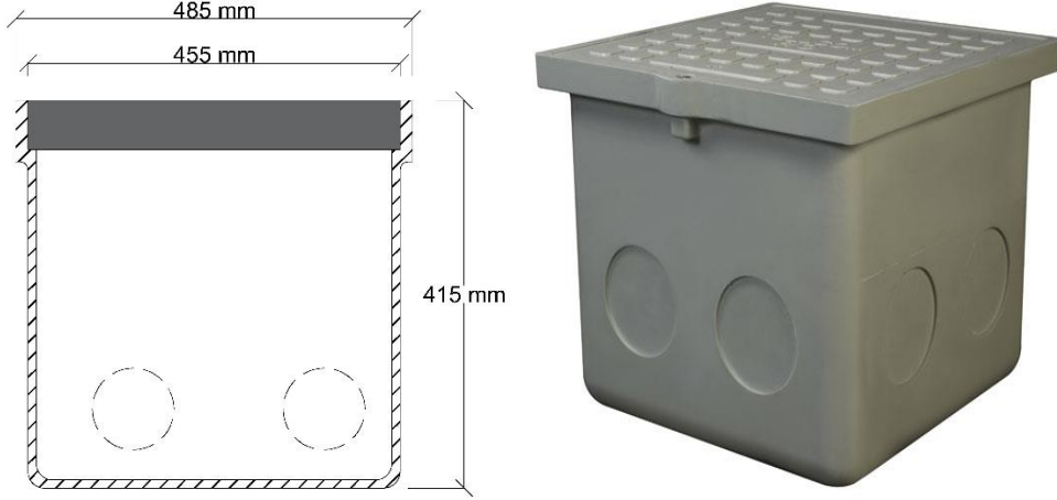
Şekil 3. TİP 10A-B Kompozit Kare Ek Odaları
