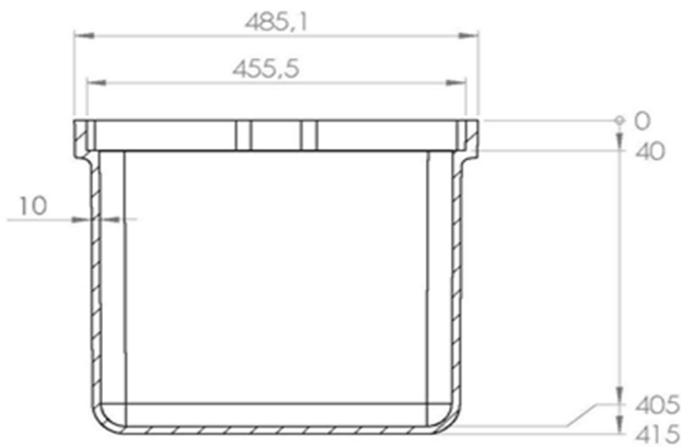
KESİT I-I ÖLÇEK 1 : 7
